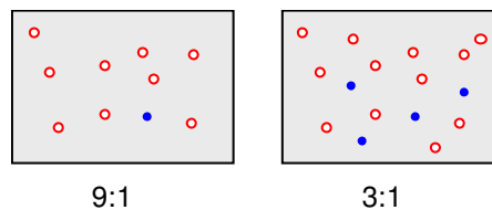
Figura 10-23. Al aumentar en cantidades iguales electrones y huecos, el aumento del portador minoritario es proporcionalmente más importante
