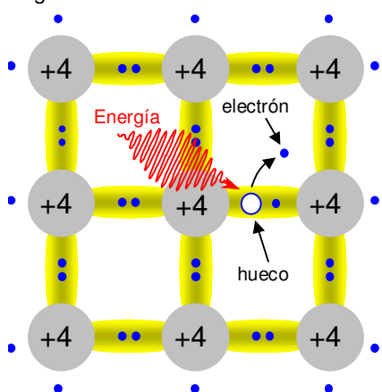
Figura 10-10. Generación de pares electrón-hueco, mediante el aporte de una determinada cantidad de energía (energía térmica, fotón, ...)
