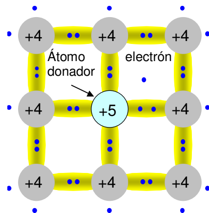
Figura 10-12. Impureza donadora en una red de silicio
