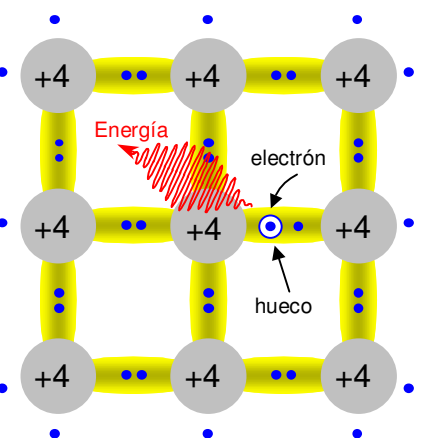
Figura 10-11. Regeneración de pares electrón-hueco, liberando una determinada cantidad de energía
