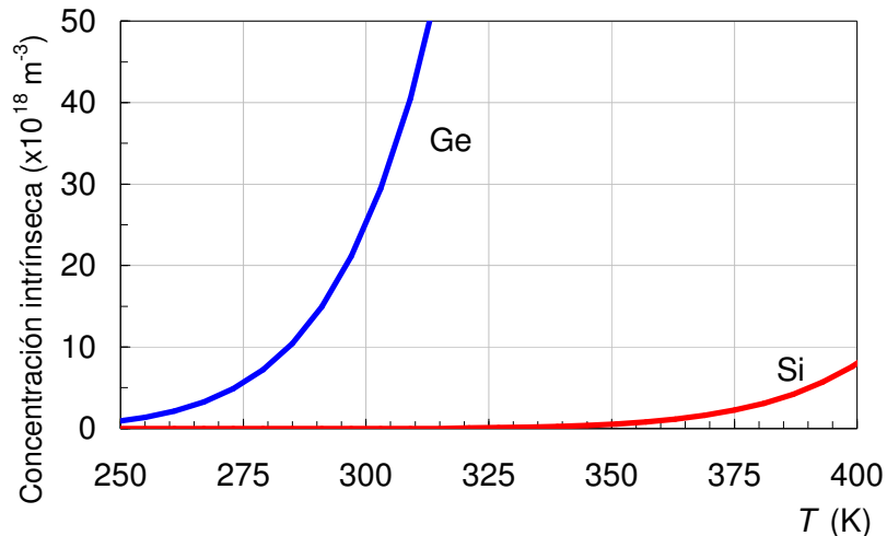
Figura 10-15. Concentración intrínseca del germanio y el silicio a distintas temperaturas
