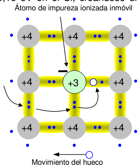
Figura 10-14. Los huecos se mueven por la caída sucesiva de electrones en ellos
