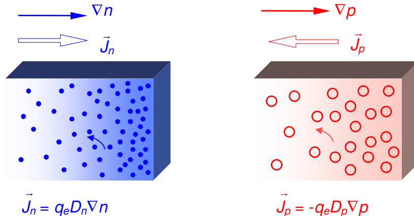
Figura 10-24. Corrientes de difusión de electrones y de huecos
