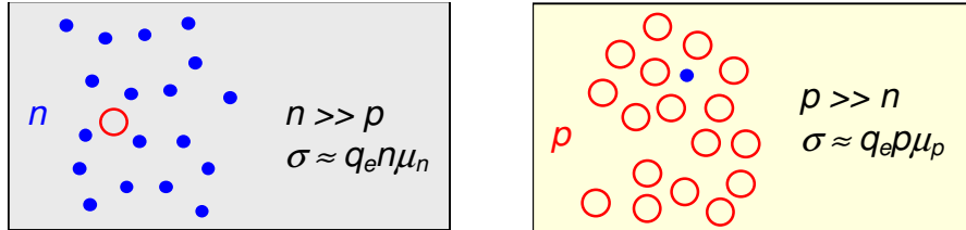
Figura 10-20. Conductividades en los semiconductores extrínsecos tipo n en la figura de la izquierda, y tipo p en la de la derecha
