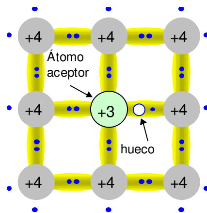
Figura 10-13. Impureza aceptora en una red de silicio
