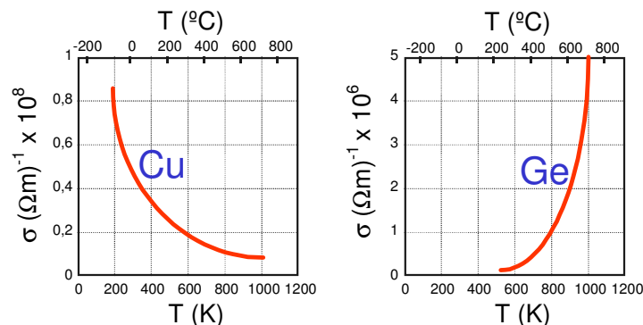
Figura 10-3. Comparación del comportamiento de conductores y semiconductores frente a la temperatura
