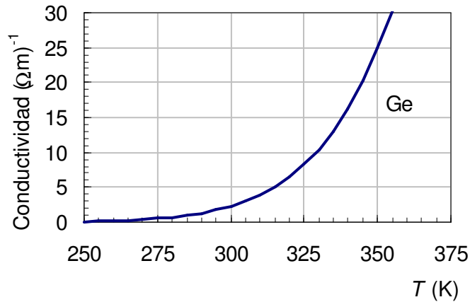
Figura 10-21. Influencia de la temperatura en la conductividad
